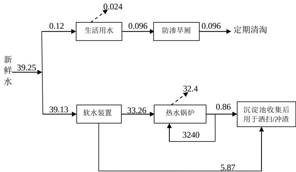
图 2 本项目水平衡图（单位：t/d）
