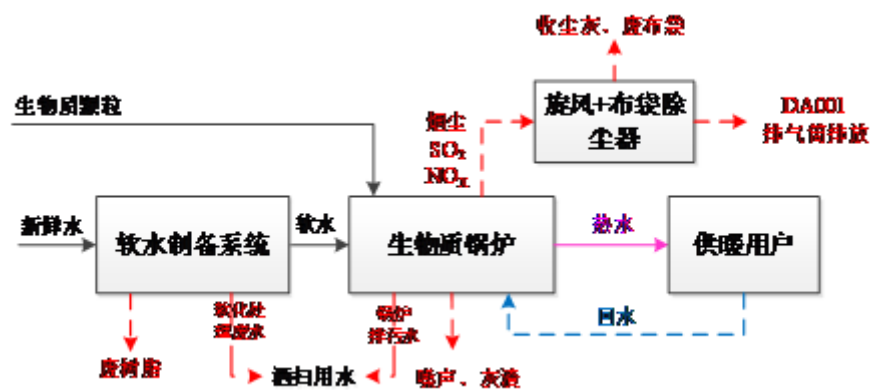
图 4 运营期工艺流程及产排污节点图
