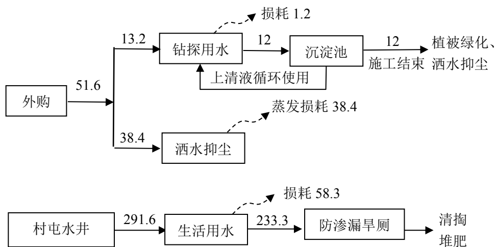
图 2-2 项目勘探期水平衡图（单位：m 3 ）
