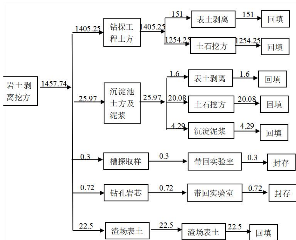
图 4-1 项目土石方平衡图（单位：m 3 ）
