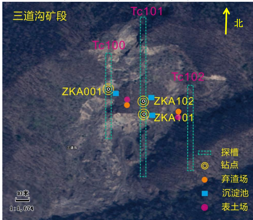
图 2-4 三道沟矿段施工平面布置示意图
