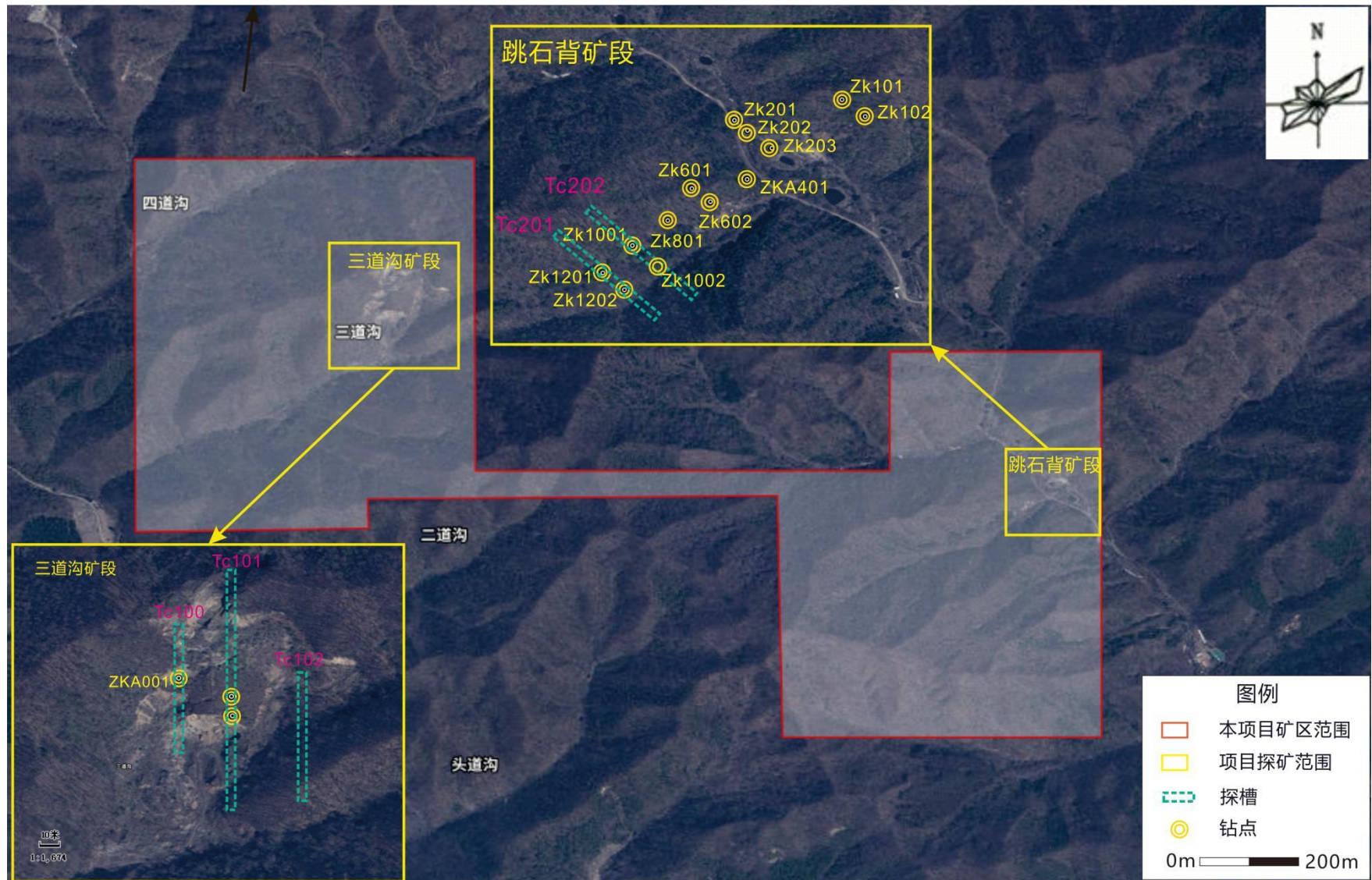
附图 8 项目探槽及探点分布图
