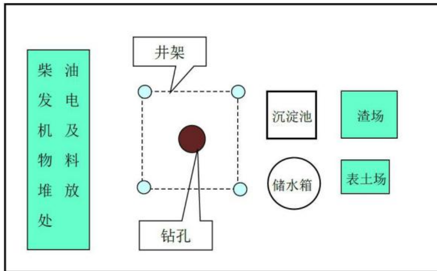
图 2-3 施工场地平面布置示意图
