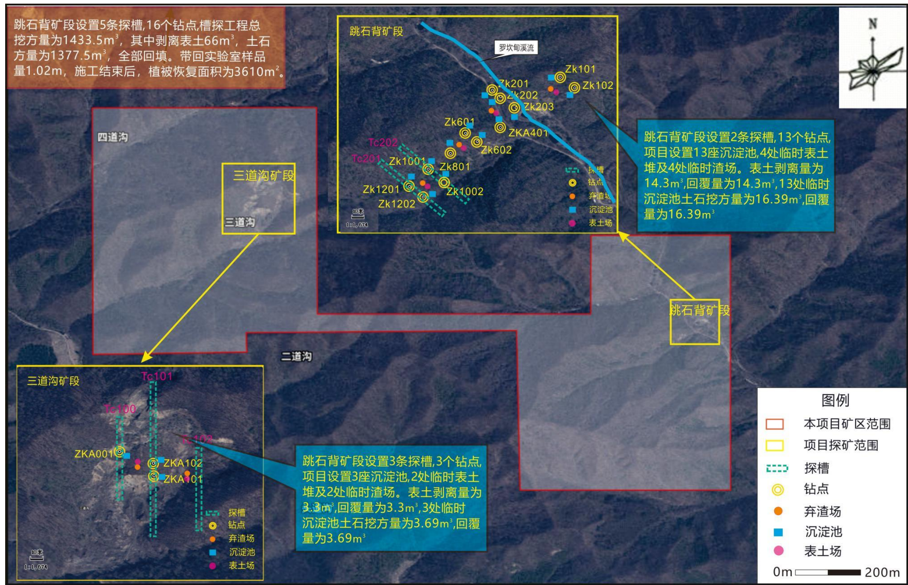
附图9 项目主要生态保护措施设计图
