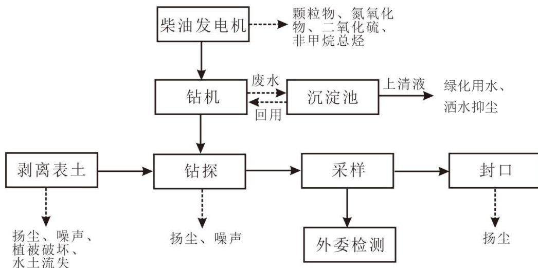
图 2-7 钻探工作工艺流程图
